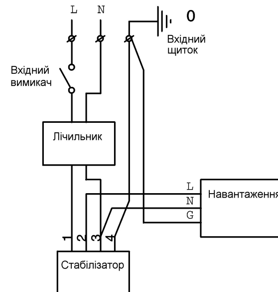
Схема підключення стабілізатора до однофазної мережі.
